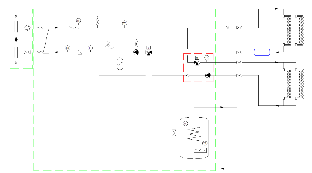
Techneco Loria Duo met 2 zone-regeling
