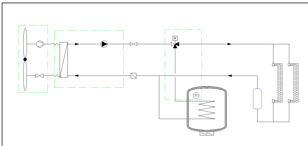
Techneco Loria met tapwaterfunctie
