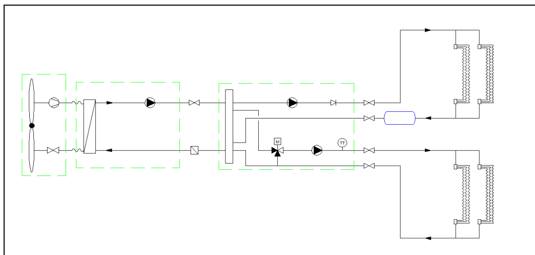
Techneco Loria met 2 zone-regeling
